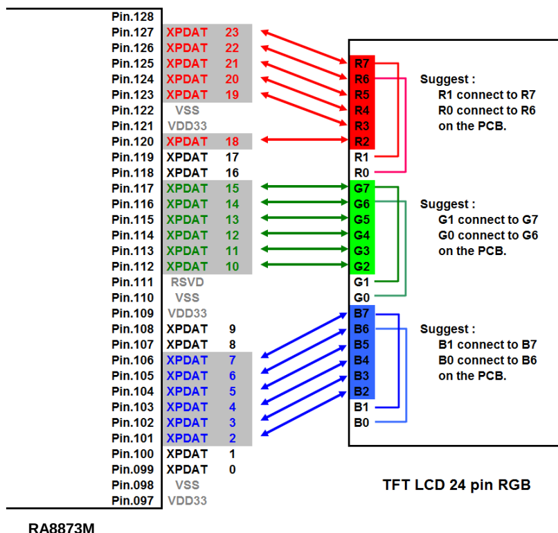
Figure 10-2 : RA8873M 色深 18bit 腳位與 LCD 螢幕腳位對應
