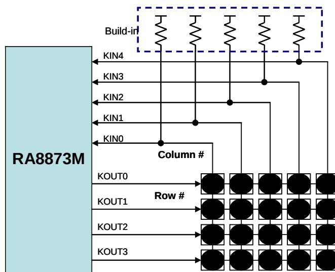
圖 17-1 : Key-Pad Application
