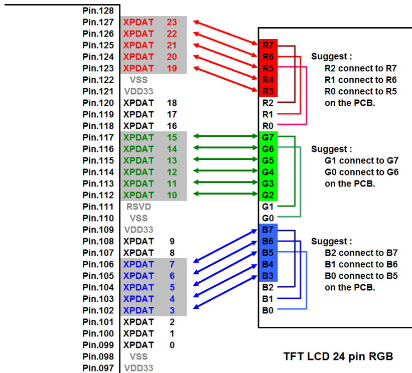
Figure 10-3 : RA8873M 色深 16bit 腳位與 LCD 螢幕腳位對應
