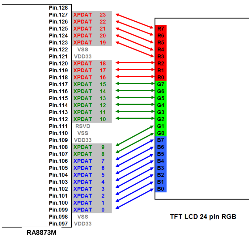
Figure 10-1 : RA8873M 色深 24bit 腳位與 LCD 螢幕腳位對應
